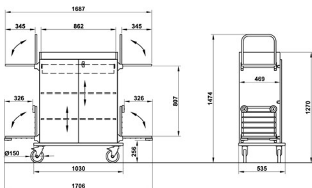
P/SE Suporte para baldes com 2 baldes
